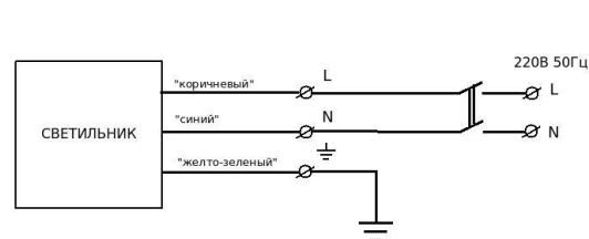
Рисунок 1. Электрическая схема подключения.
